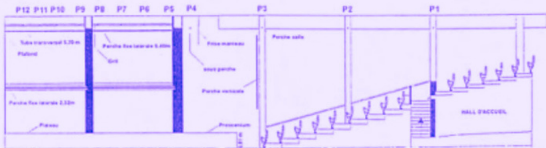
FIG.c COUPE SCÈNE/SALLE
