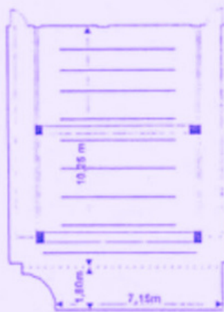
FIG.b PLAN PLATEAU PROSCENIUM
